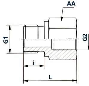
Uzun Tip / Long Type
