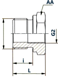
Kısa Tip / Short Type
