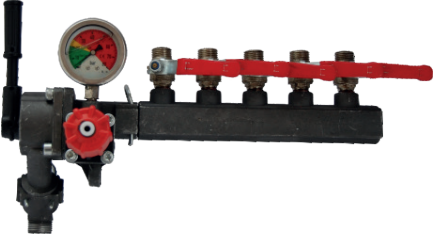
VDR 50 Regülatör 5'li Çıkış VDR 50 Regulator 5 Output
